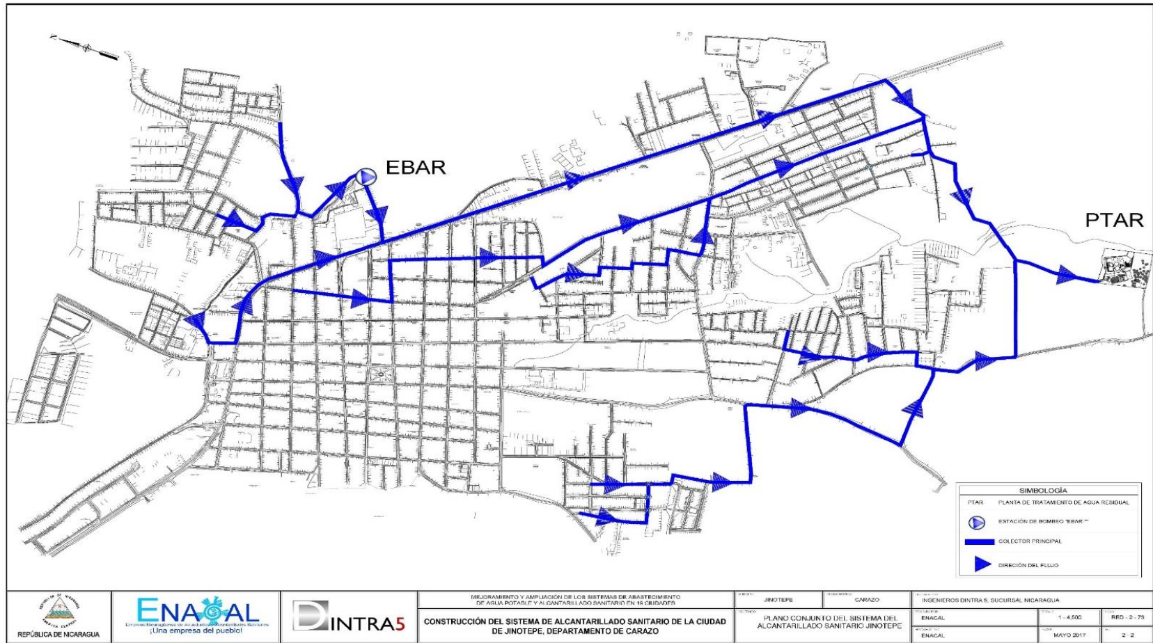
Esquema del mejoramiento y ampliación del Sistema de Alcantarillado Sanitario y Tratamiento de Aguas Residuales de Jinotepe, Carazo.
